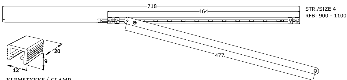
KLEMSTYKKE / CLAMP
